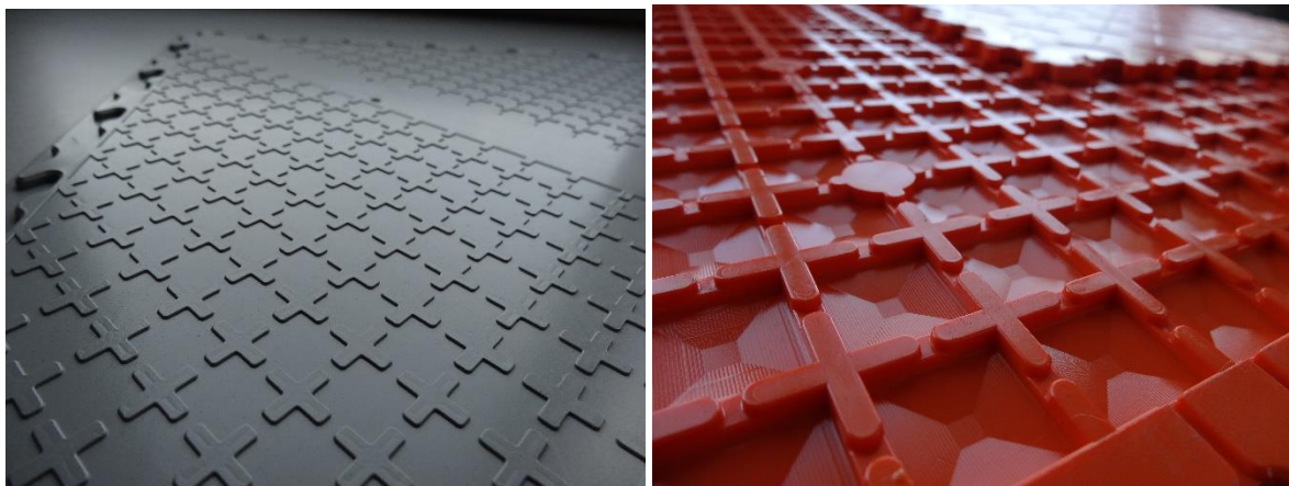
System AirFlow płytek Fortelock Invisible i Fortelock Light
