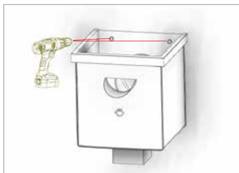
rys.3 Wykonanie otworów pod kołki w tylnej ścianie kosza zlewowego.
