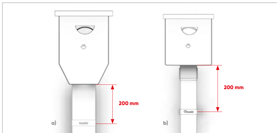
rys.8 Połączenie pionu spustowego do ściany a) system STAL, b) system STAL².
